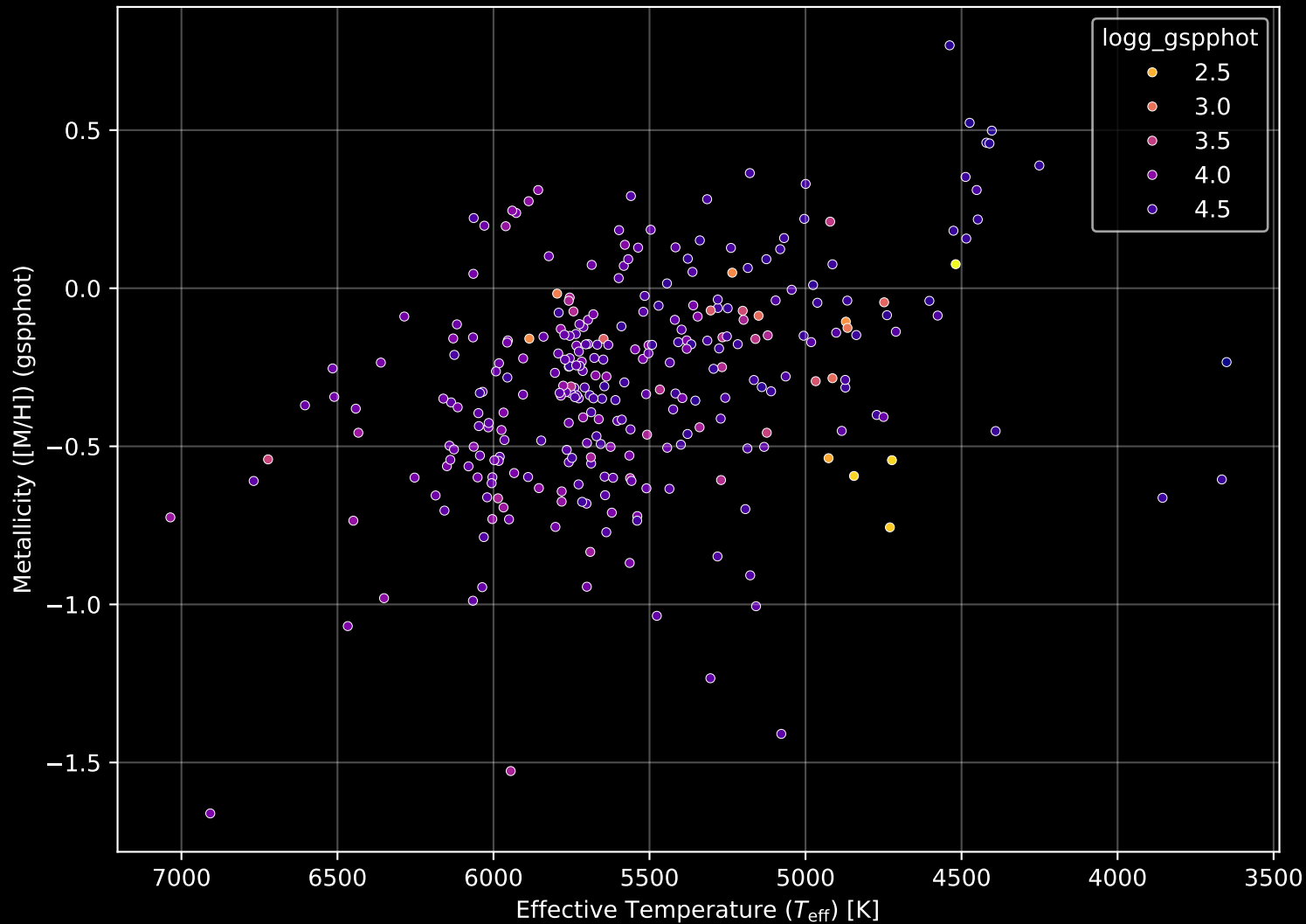
GALAH DR4 Field: [7063] Stellar Population Parameters (n= 296)
