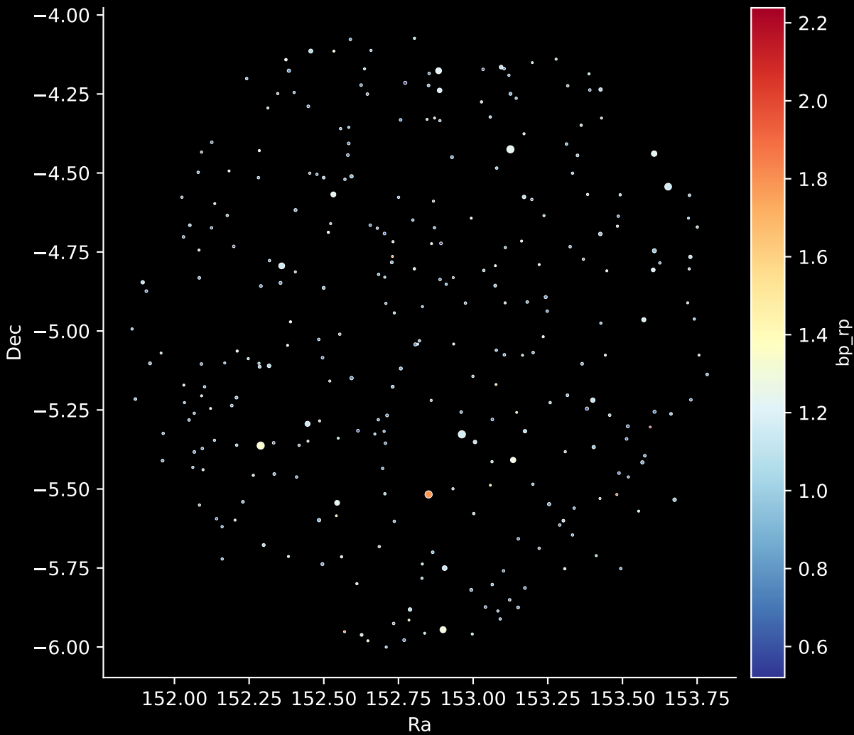
GALAH DR4 Field: [7063] Stars: 296
