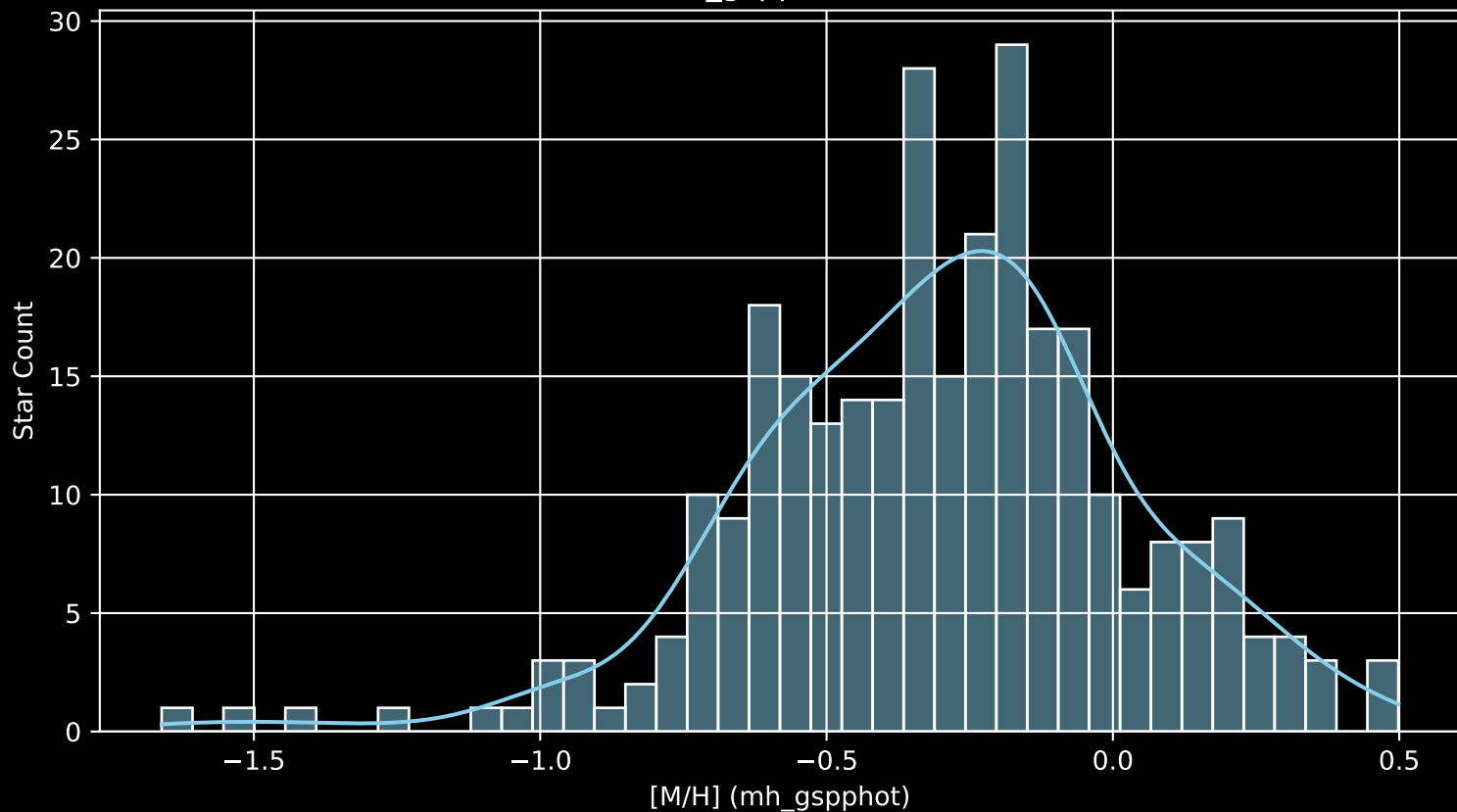
GALAH DR4 Field: [7063] [M/H] (mh_gspphot) (n= 294)
